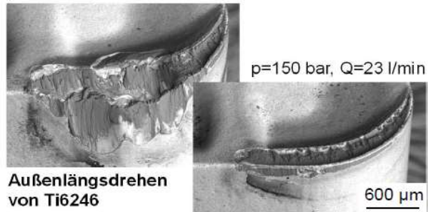
Werkzeugverschleiß mit HD-KSS-Zufuhr
